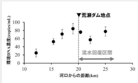
中央/ダム撤去によってよみがえった瀬。 2017年8月の調査ではDNA量が最も大きかった。 左/DNA抽出作業。 下/図 球磨川における河川水中のアユの環境DNA濃度。
