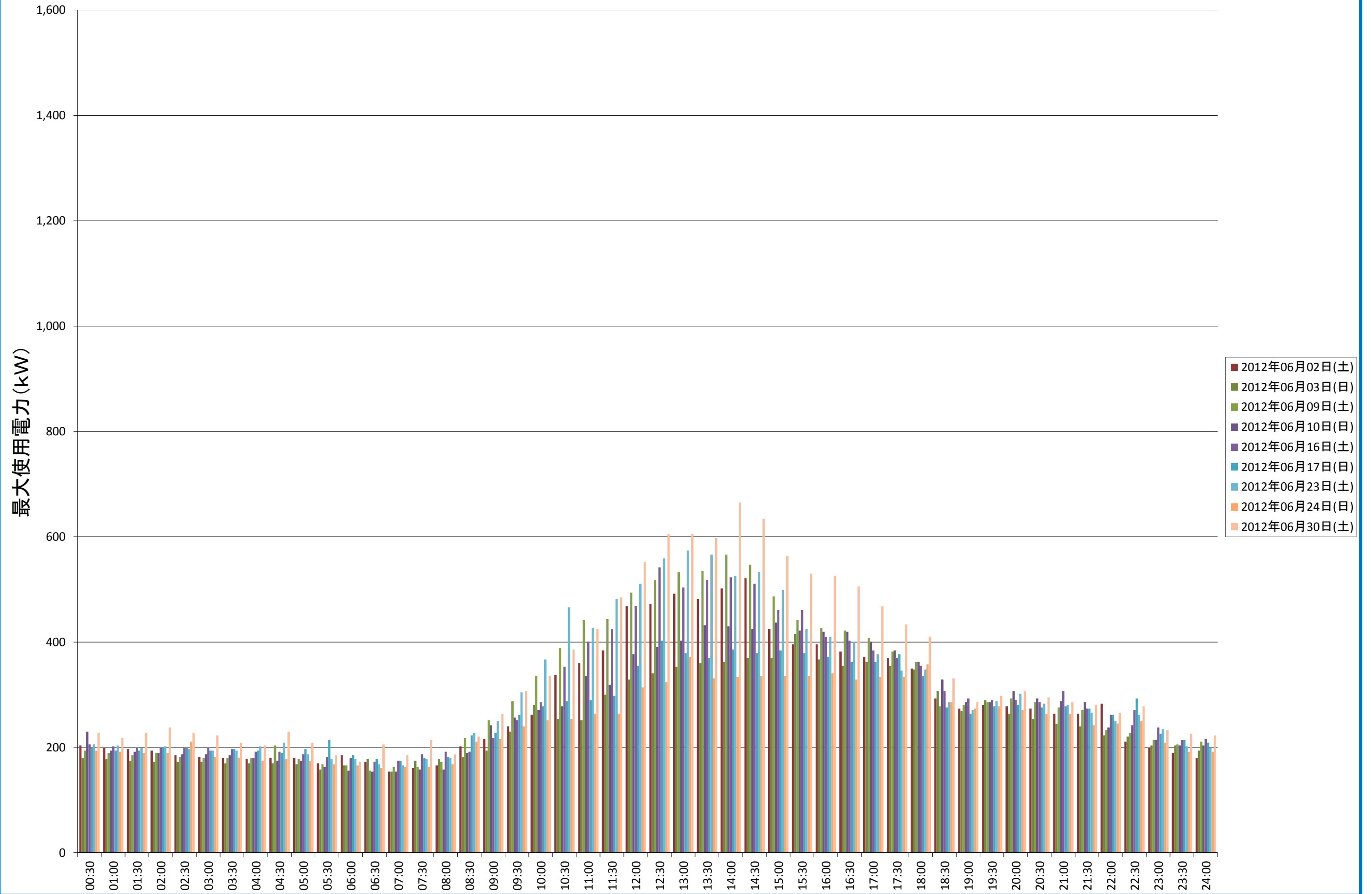
黒髪北キャンパス 6月の時間帯別最大使用電力(土日祝)
